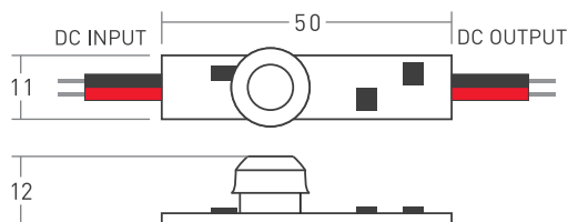
Рисунок 1. Габаритные размеры выключателя SMART-MOTION
